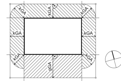
Kleiner und grosser Grenzabstand
