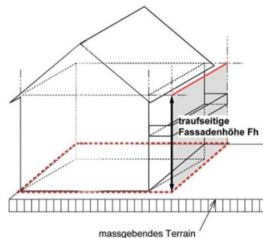
Abbildung: Neue Messweise der zulässigen Fassadenhöhe traufseitig F_{h\ tr}
