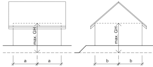
Abbildung: Bisherige Messweise der zulässigen Gebäudehöhe
